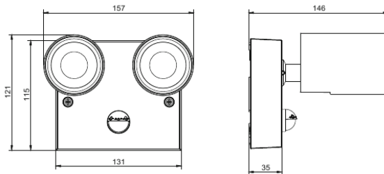
W157 x H121 x D146mm
